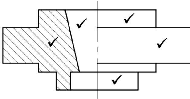
FLANGE - ITEM 5
