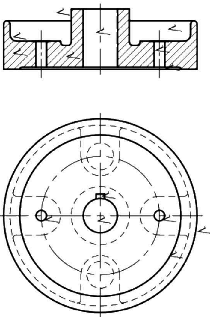
THE FLANGE (ITEM 1A)✓
