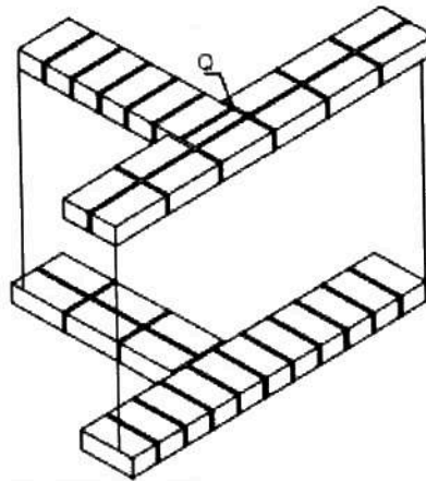
'N T-AANSLUITING VAN TWEE EENSTEENMURE IN ENGELSE VERBAND
