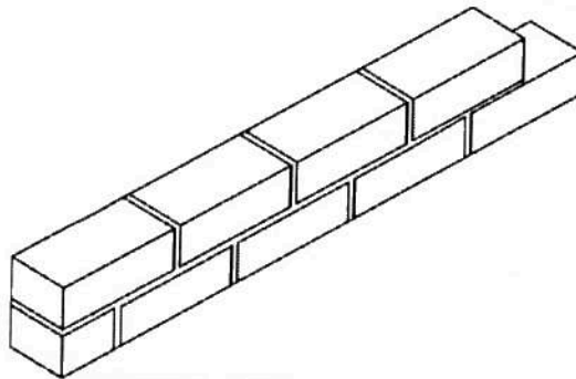
HALFSTEENMUUR IN STRYKVERBAND
