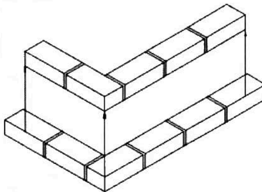
HOEKAANSLUITING VAN TWEE HALFSTEENMURE IN STRYKVERBAND
