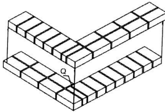
HOEKAANSLUITING VAN TWEE EENSTEENMURE IN ENGELSE VERBAND
