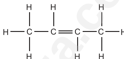
but-2-ene
