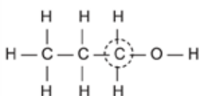
propaan-1-ol
