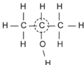
propaan-2-ol
