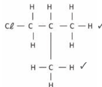
1-chloor-2-metielpropaan
