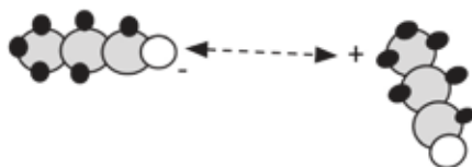
'n Voorbeeld van dipool-dipool-kragte tussen twee propaanaalmolekule
