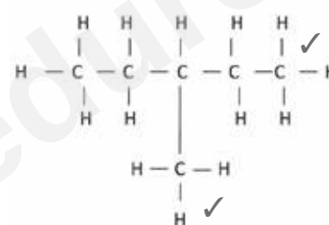
3-metielpentaaan
