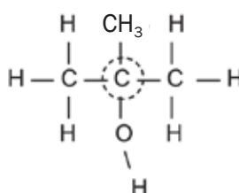
metiel propaan-2-ol
