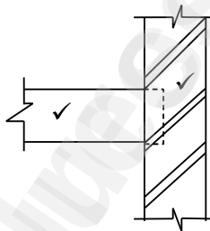
Vloerbalk in die muur ingebou
