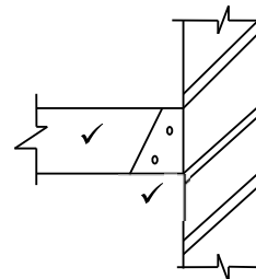
Vloerbalk met 'n aanhanger aan die muur gebout
